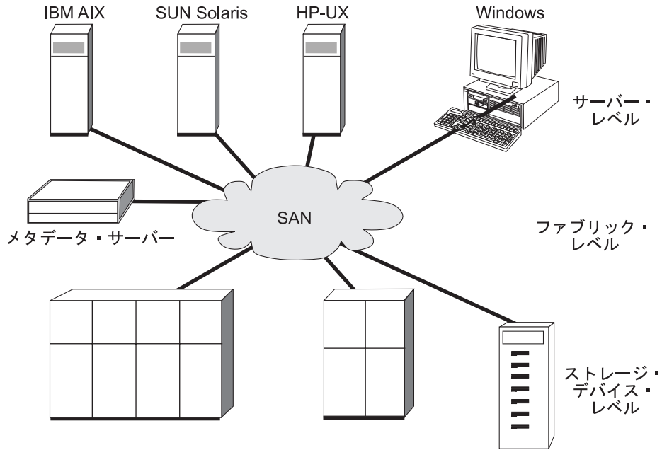
図1. バーチャリゼーションのレベル
