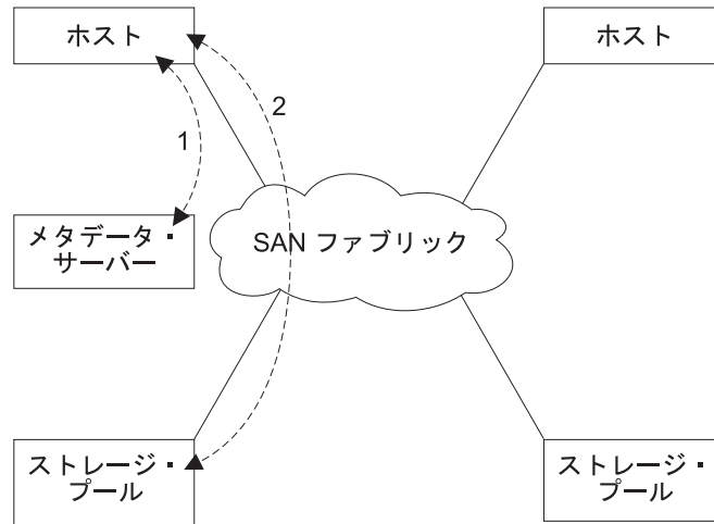
図2. 非対称バーチャリゼーション
