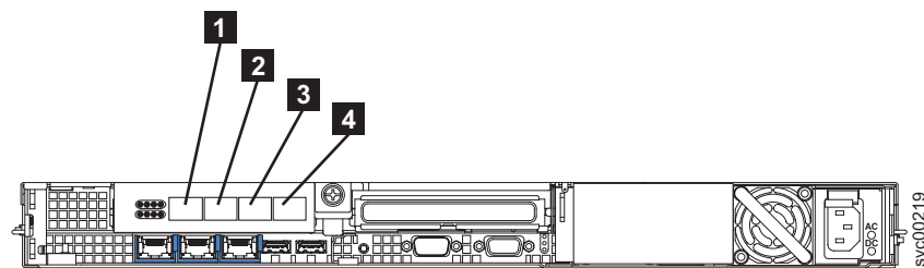
図 24. SAN ボリューム・コントローラー 2145-8G4 の物理ポート番号
