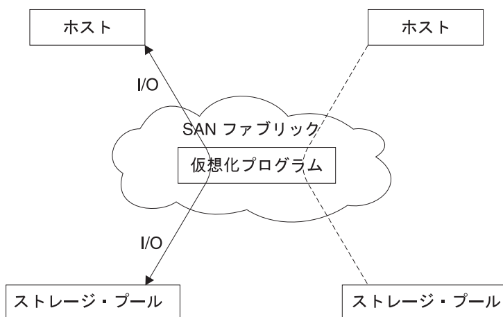
図3. 対称バーチャリゼーション
