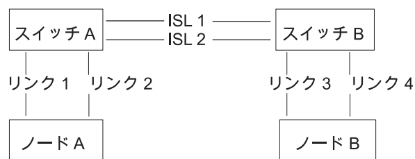
図 16. クラスタ内のノード間でスイッチ間リンクがあるファブリック
