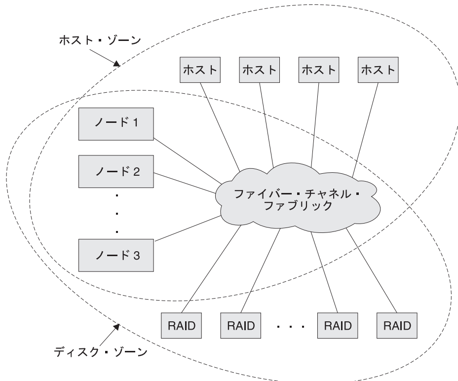
図 12. ファブリック内の SAN ボリューム・コントローラー の例
