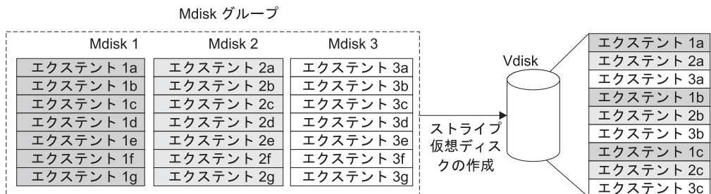
図 9. MDisk グループと VDisk
