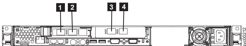
図 26. SAN ボリューム・コントローラー 2145-8F2 の物理ポート番号
