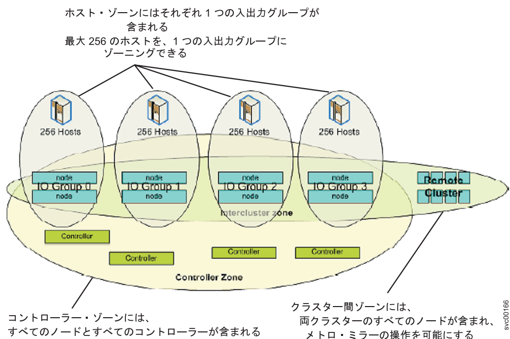
図 18. 1024 ホスト構成のゾーニング
