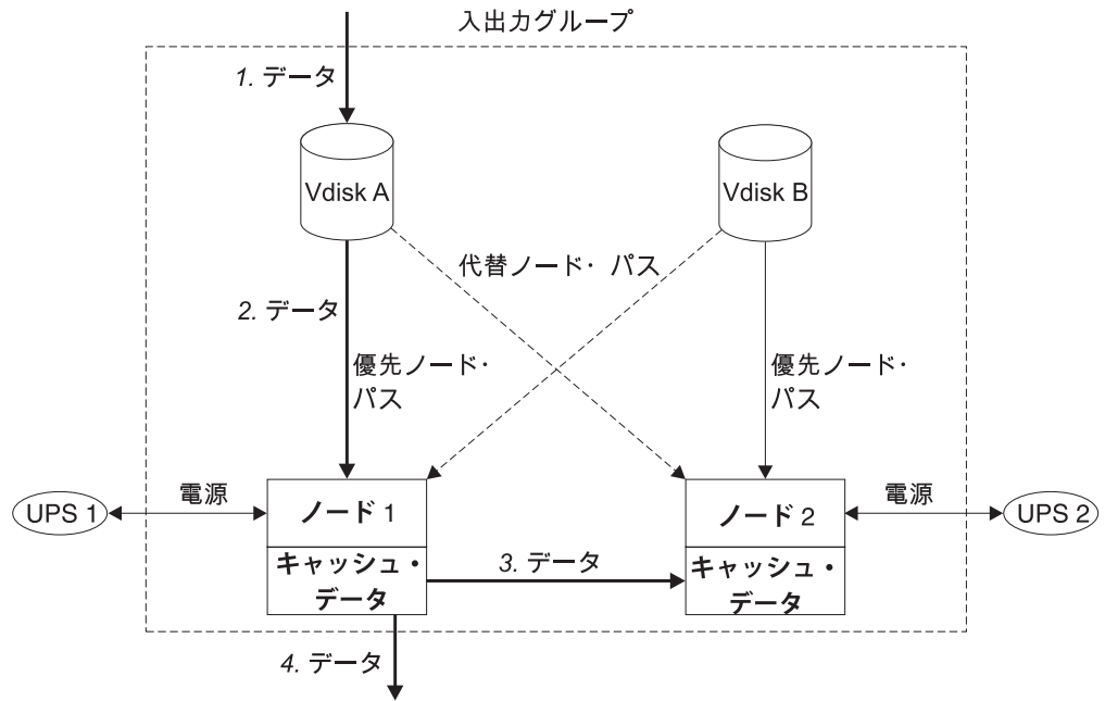
図6. 入出力グループと UPS
