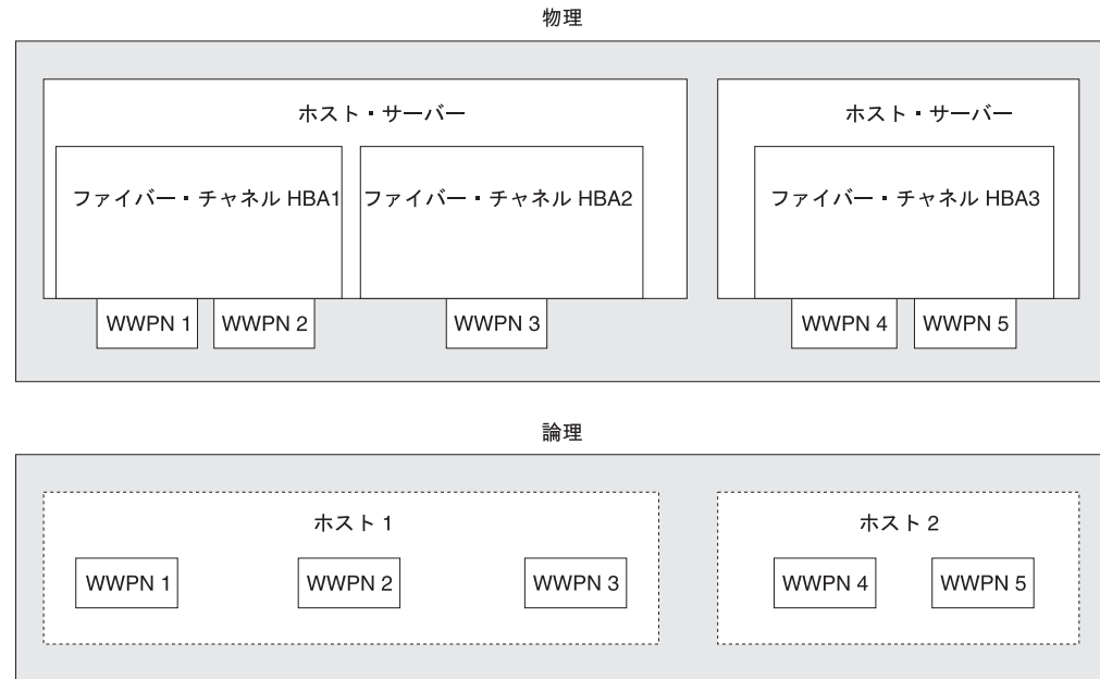
図 10. ホスト、WWPN、および VDisk
