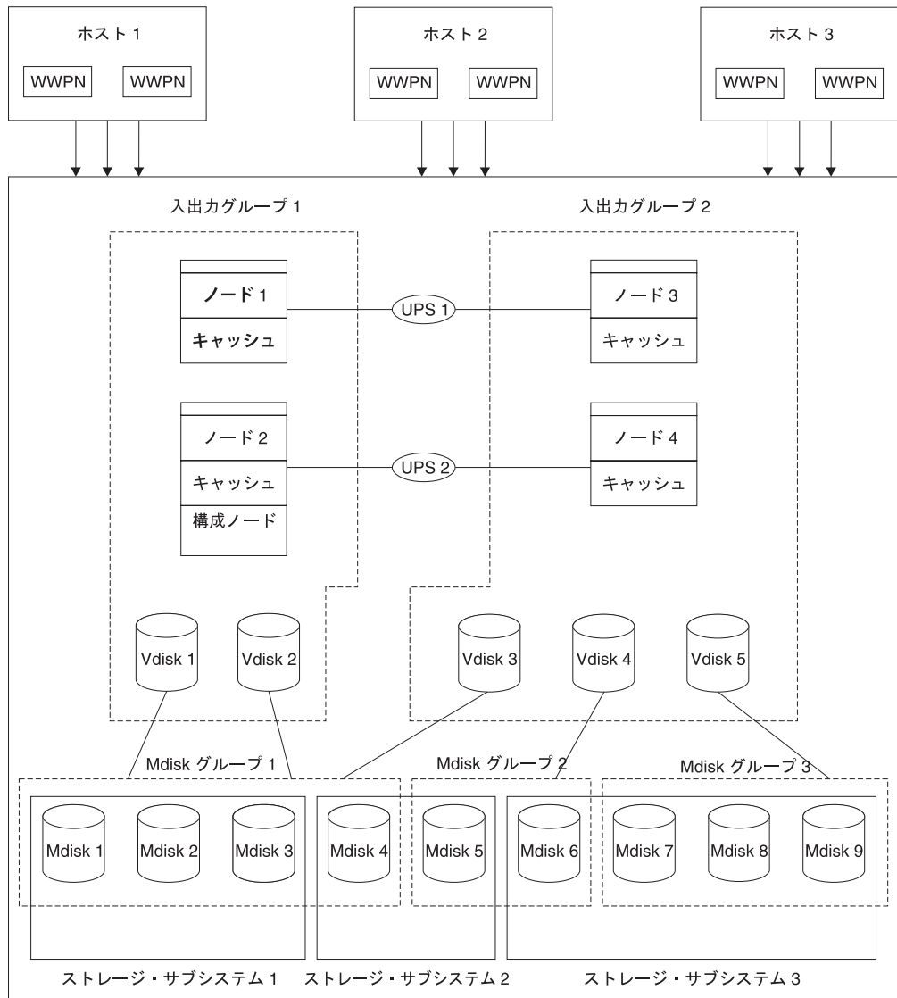
図 4. バーチャリゼーション
