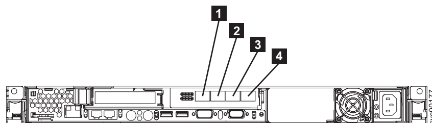
図 25. SAN ボリューム・コントローラー 2145-8F4 の物理ポート番号
