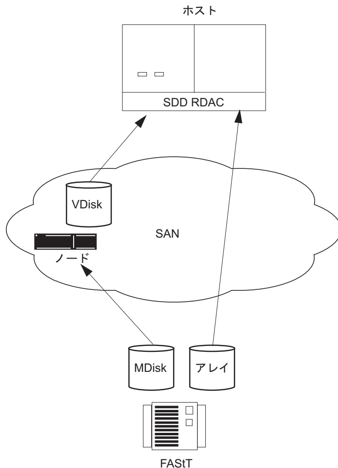
図 16. 1 つのホスト上で SAN ポリリューム・コントローラー・ノードを使用する IBM DS4000 直接接続
