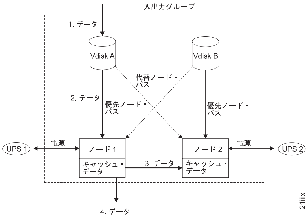
図 5. 入出力グループと無停電電源装置
