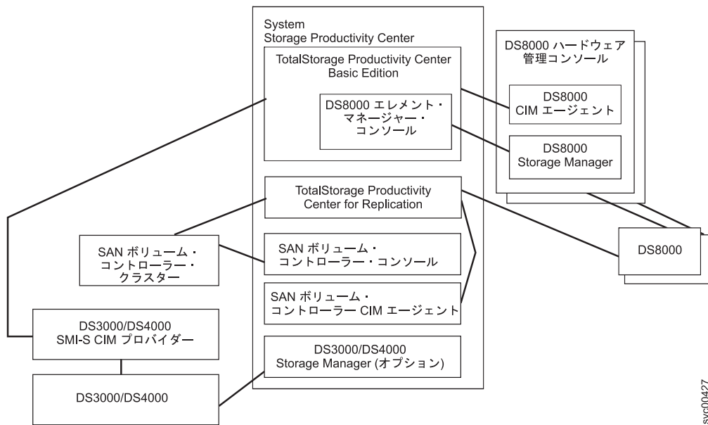
図 11. IBM System Storage Productivity Center の概要
