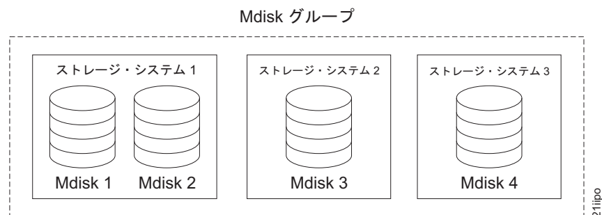
図 7. MDisk グループ
