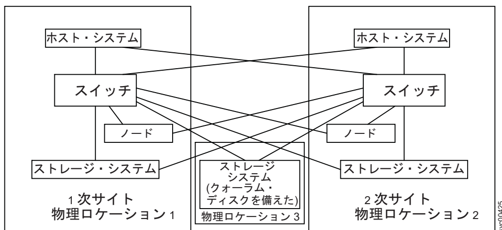
図 25. クォーラム・ディスクを使用した有効な分割クラスター構成
