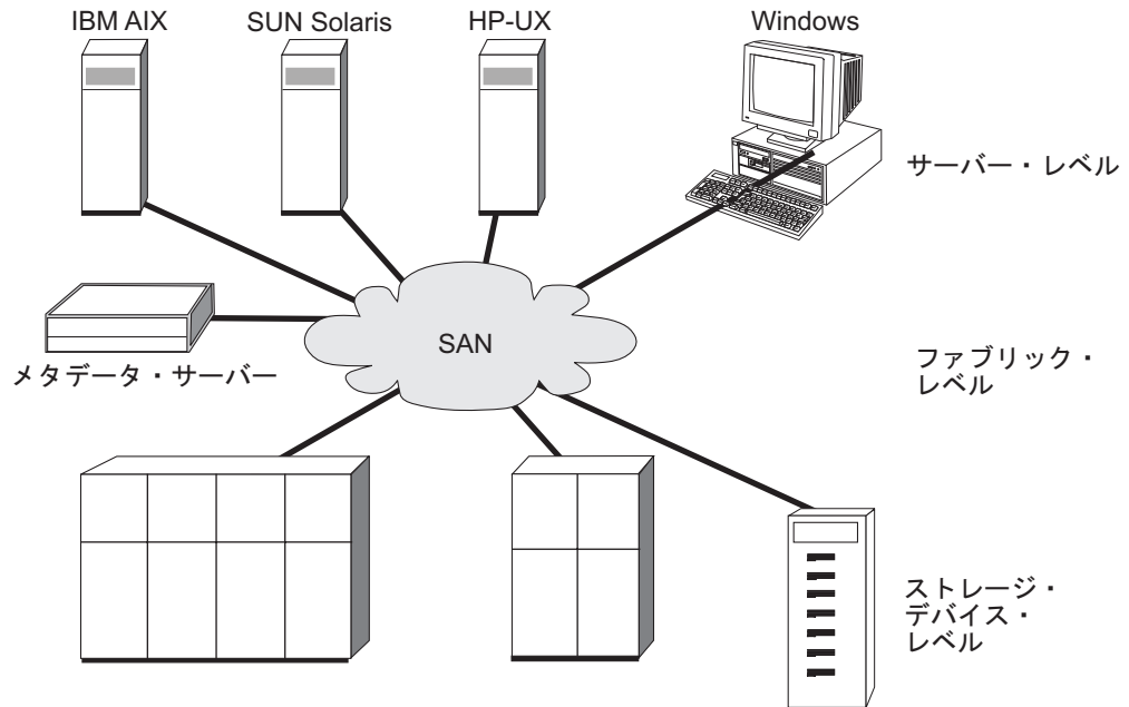
図1. 仮想化のレベル
