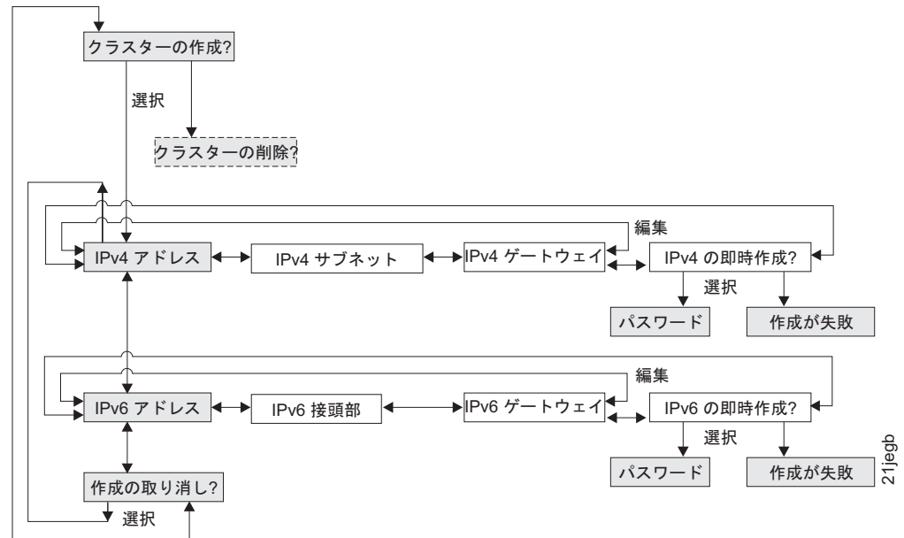
図 26. クラスターの作成? ナビゲーション
