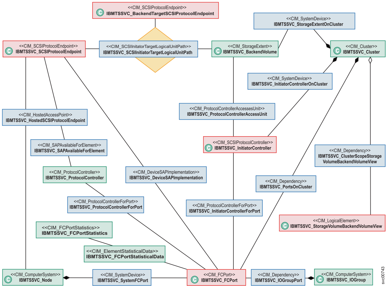
图 16. FC 端口实例的类图
