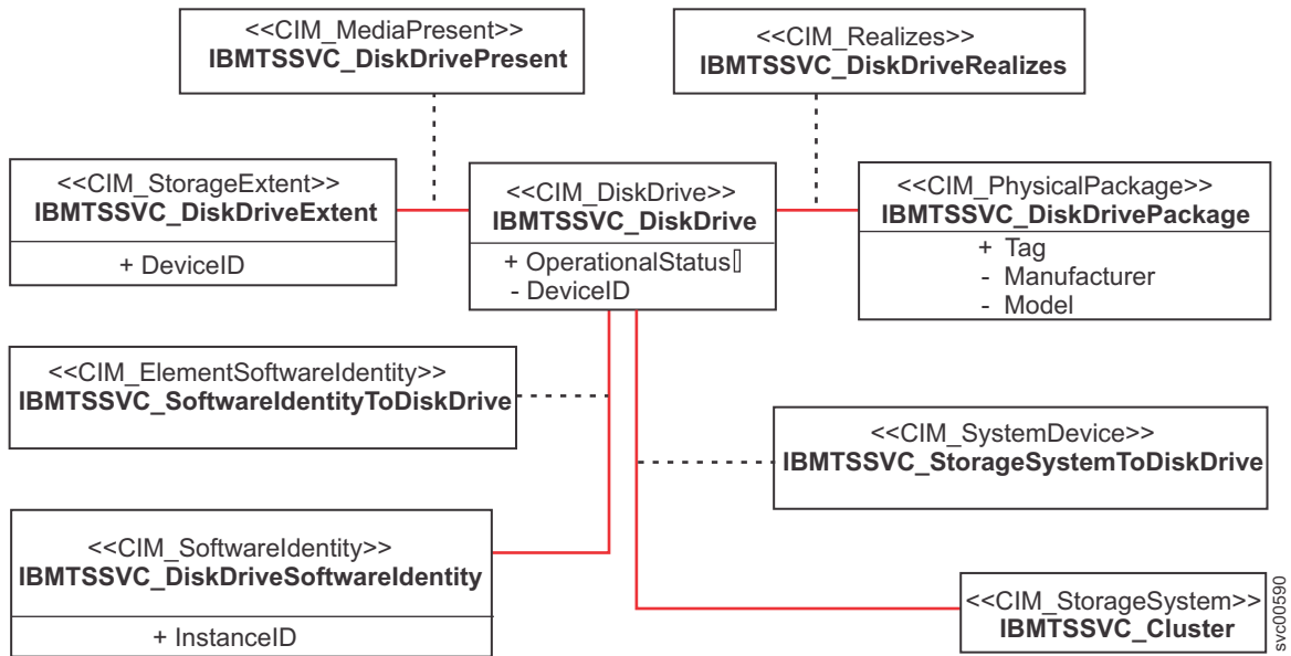
图 10. 磁盘驱动器 Lite 概要文件的统一建模语言元素概述
