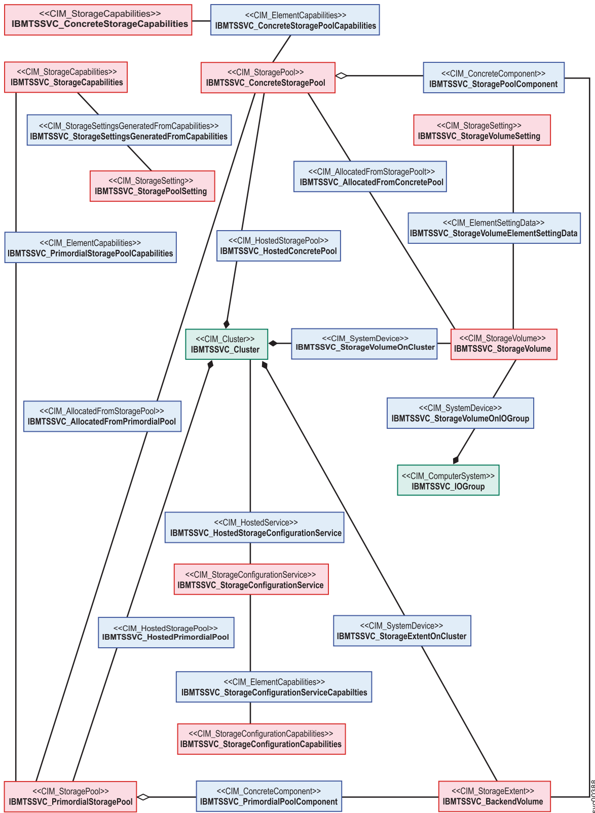
图 6. 块服务的高级概述。
