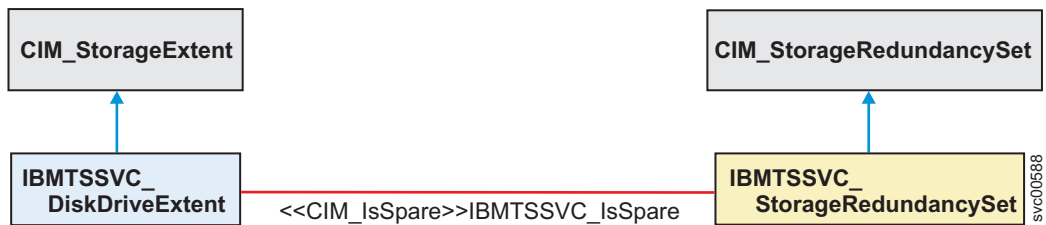
图 12. IsSpare 关联
