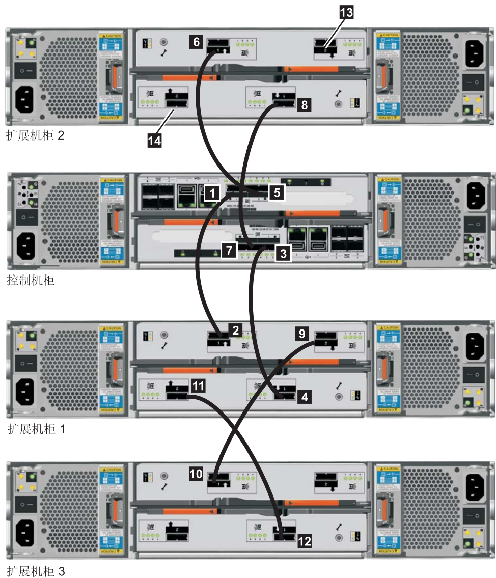
图 14. 将 SAS 电缆连接到机柜
