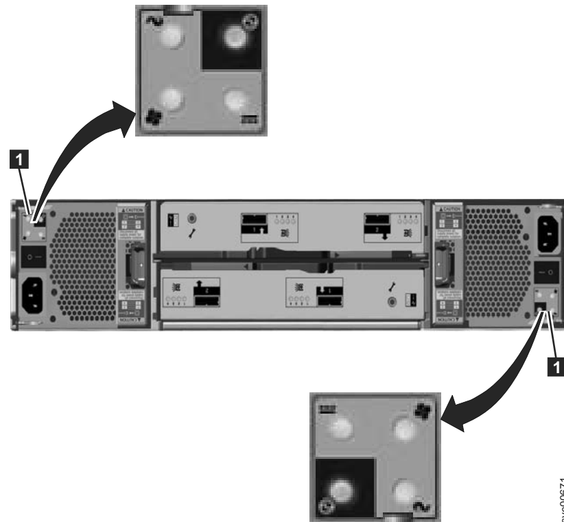
图 16. 扩展机柜电源单元上的指示灯
