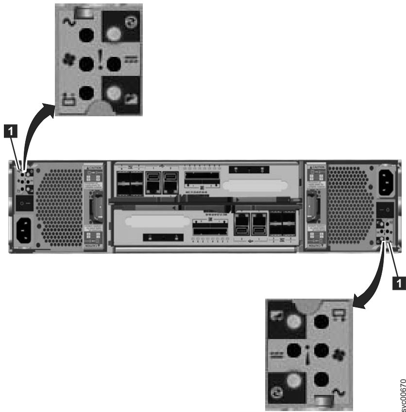
图 17. 控制机柜电源单元上的指示灯
