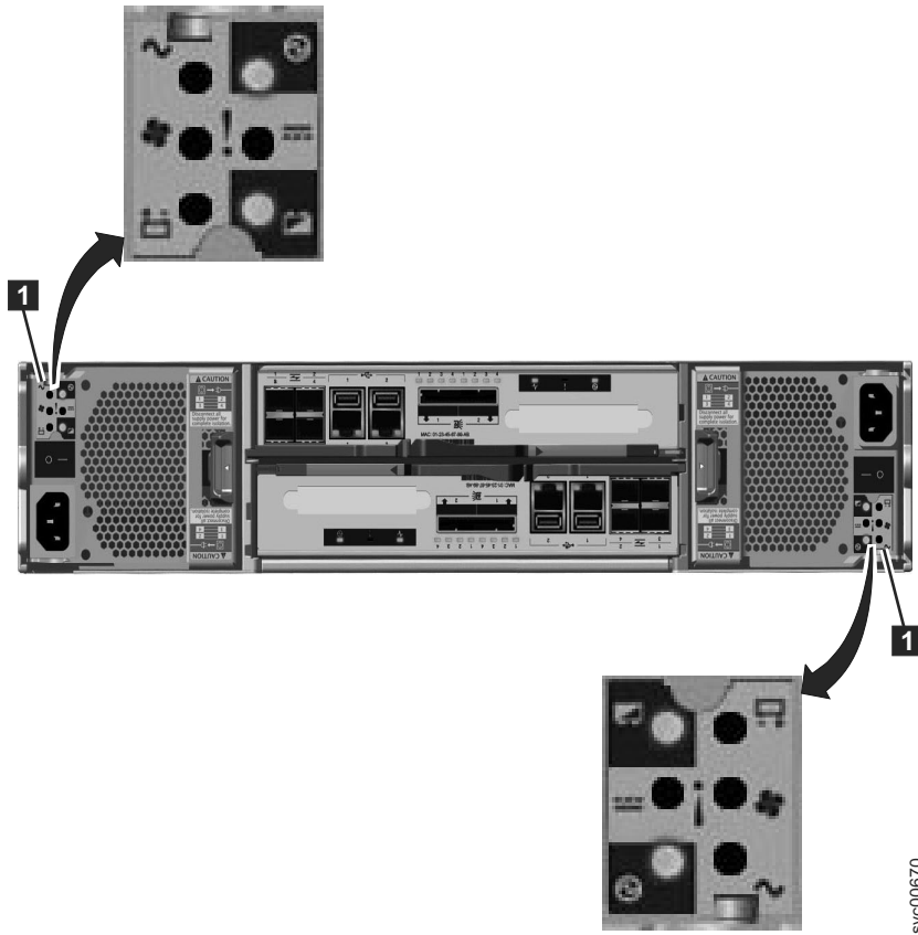
図 17. コントロール・エンクロージャの電源機構装置上の LED
