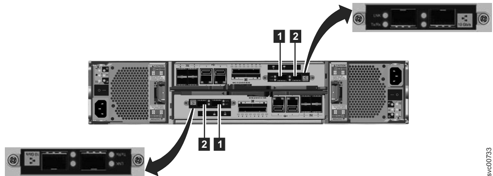
図 5. Storwize V7000 エンクロージャーの背面にある 10 Gbps イーサネット・ポート
