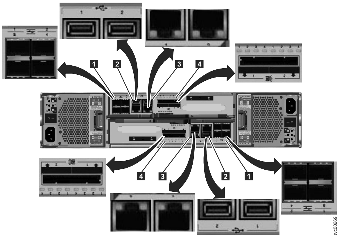
図 4. コントロール・エンクロージャーの背面のデータ・ポートおよび LED
