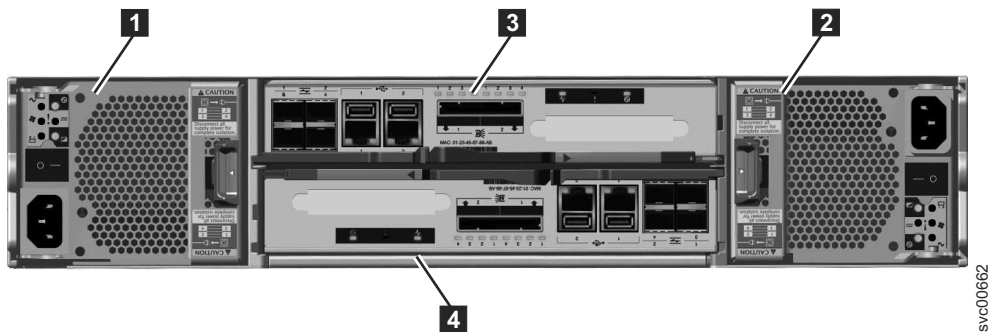
図3. モデル 2076-112 またはモデル 2076-124 コントロール・エンクロージャーの背面図
