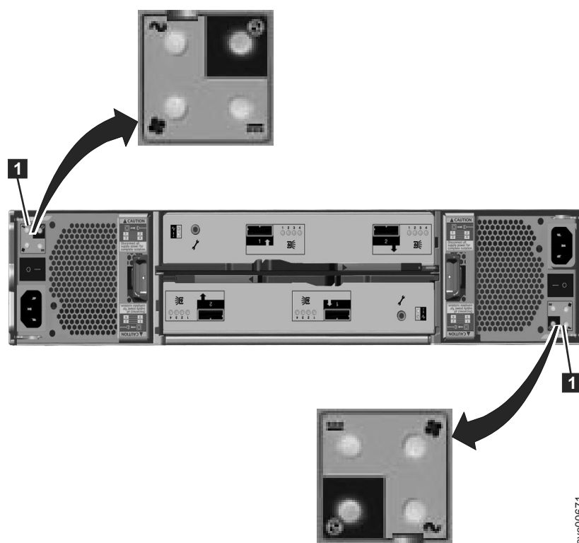
図 16. 拡張エンクロージャの電源機構装置上の LED
