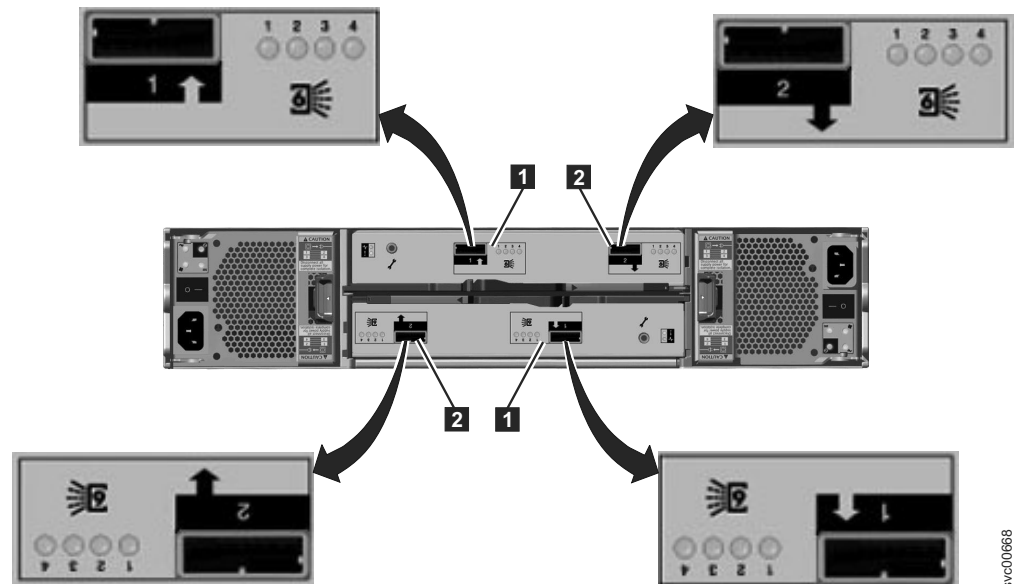
図7. 拡張エンクロージャの背面の SAS ポートおよび LED
