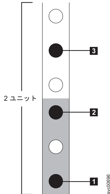
図9. ラックの背面のホール位置
